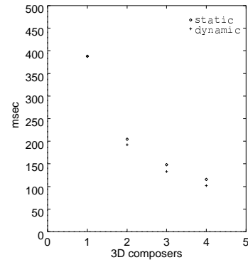
図 13 分割方法の変更による実行フェーズにかかる時間の短縮 Fig. 13 Reduction of execution phase time by changing the division method.
