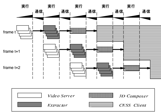
図6 パイプラインの構成 Fig. 6 Pipeline structure.
